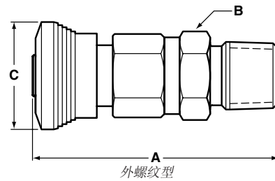
外螺纹型
