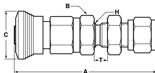
穿板卡套型 如需 'H' 和 'T' 尺寸, 请参阅第 6 页
